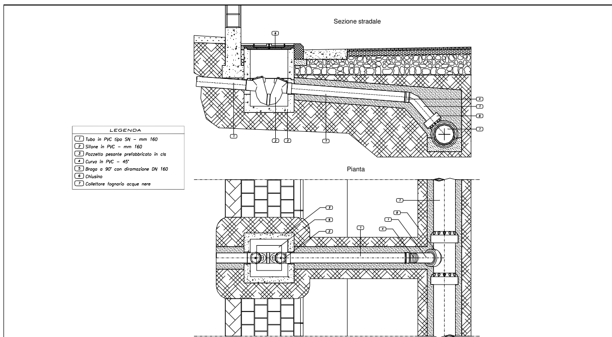
Figura 3. Allaccio tipo
